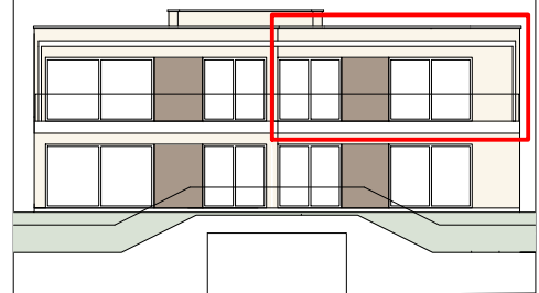
SÜDANSICHT
